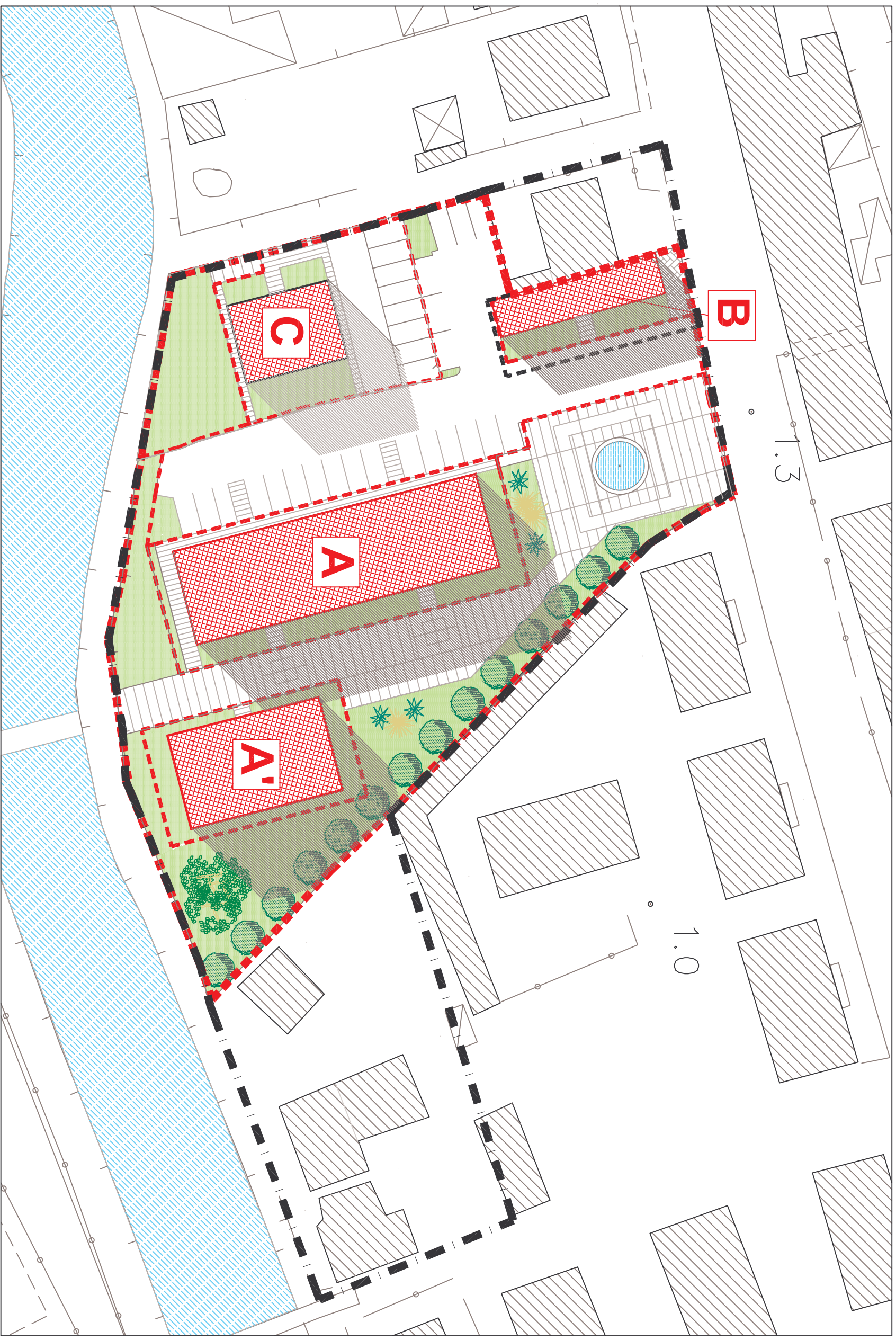
COMPARTI 1 e 2 - Planivolumetrico 1:500
